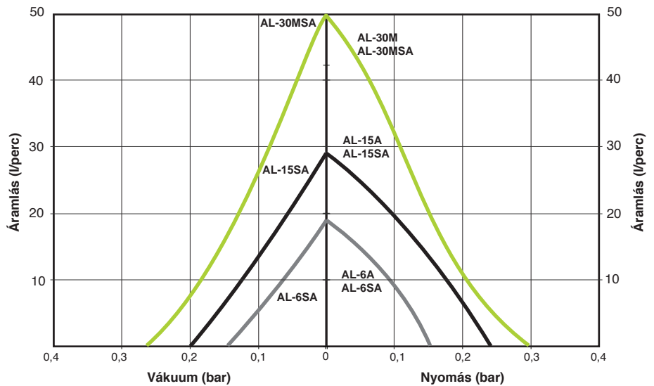
Nyomás és vákuum modellek AL-6SA, AL-15SA, AL-30MSA
